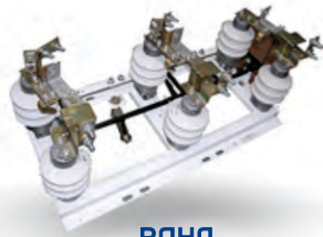
РПНД РАЗЪЕДИНИТЕЛИ 10 КВ
