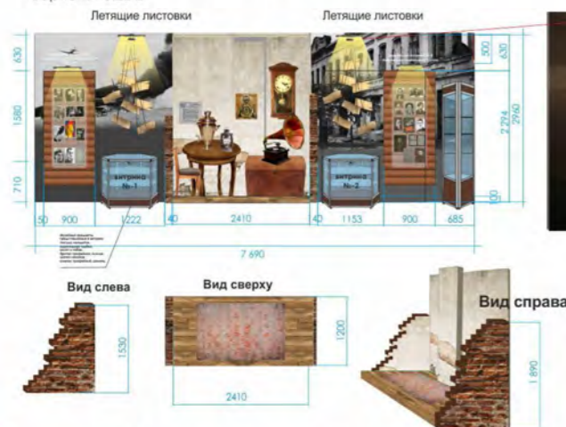
РАЗВЕРТКА 1-2 по оси В с размерами (ВИТРИНА № 1,2) Вариант - 5.2E-2
