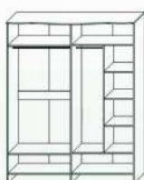
Шкаф для одежды «4Д Стефани» КМК 0649.3 1830*2200*600
