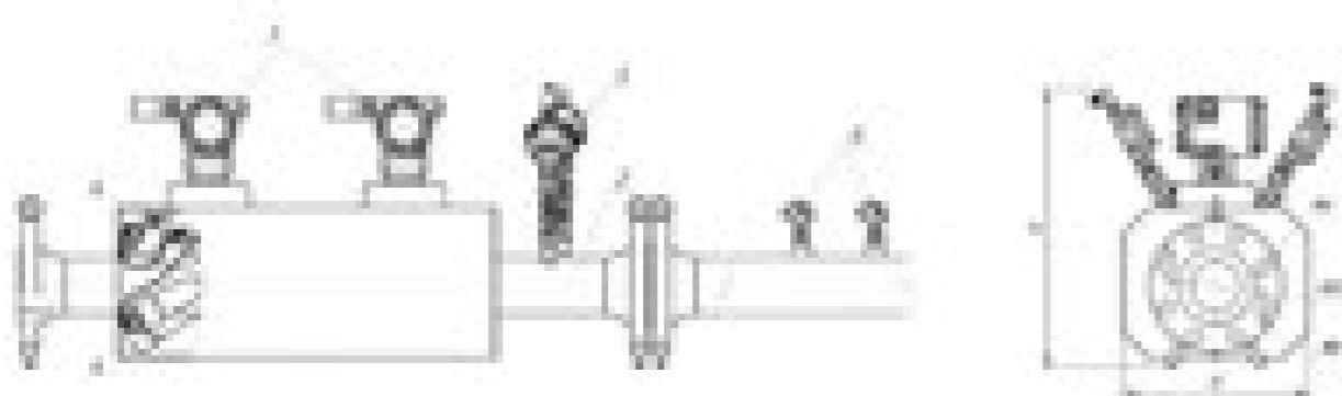
Габаритные размеры расходомера. Исполнение корпуса с дублированием – dA
